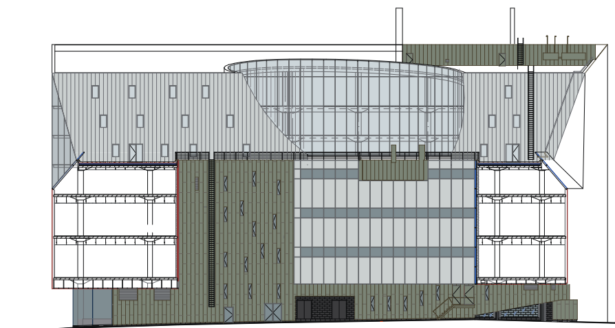
Elevations / 立面图
