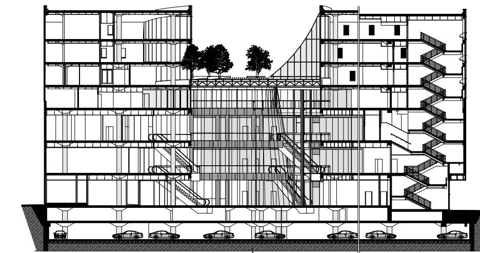
Sections / 切面图
