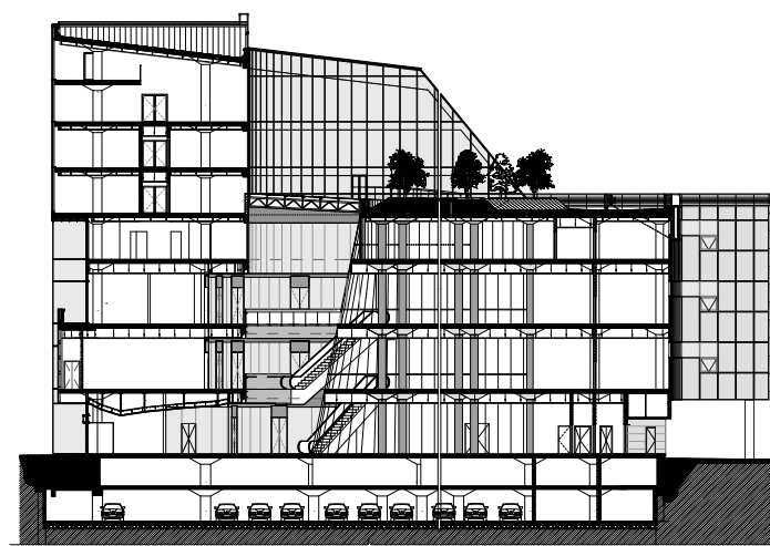
Sections / 切面图
