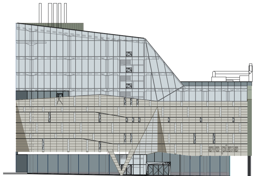
Elevations / 立面图
